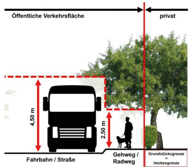
Das Lichtraumprofil zeigt an, wie weit die Bepflanzung zurückgeschnitten werden muss.
